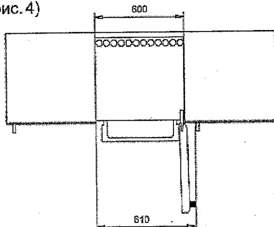
Рис. 4 Вид сверху
